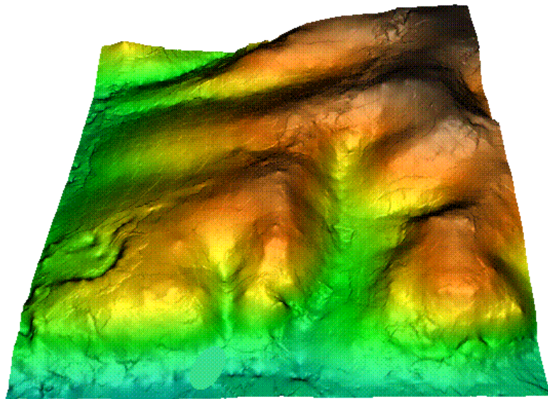
Kriging
